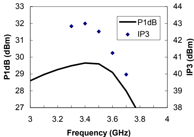
V ds =5V, I ds =0.5 I dss , Test CKT @ 3.5 GHz
